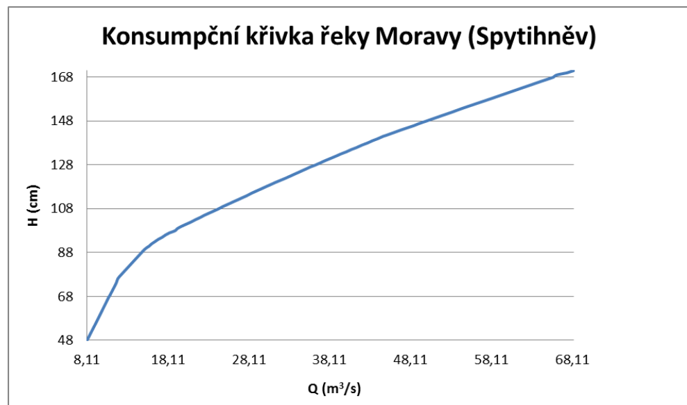
Obrázek 37 Konzumpční křivka řeky Moravy v profilu Spytihněv sestavená z dat pro říjen 2012 (seminární práce studentů – autorka O. Škrabalová, 2012)
