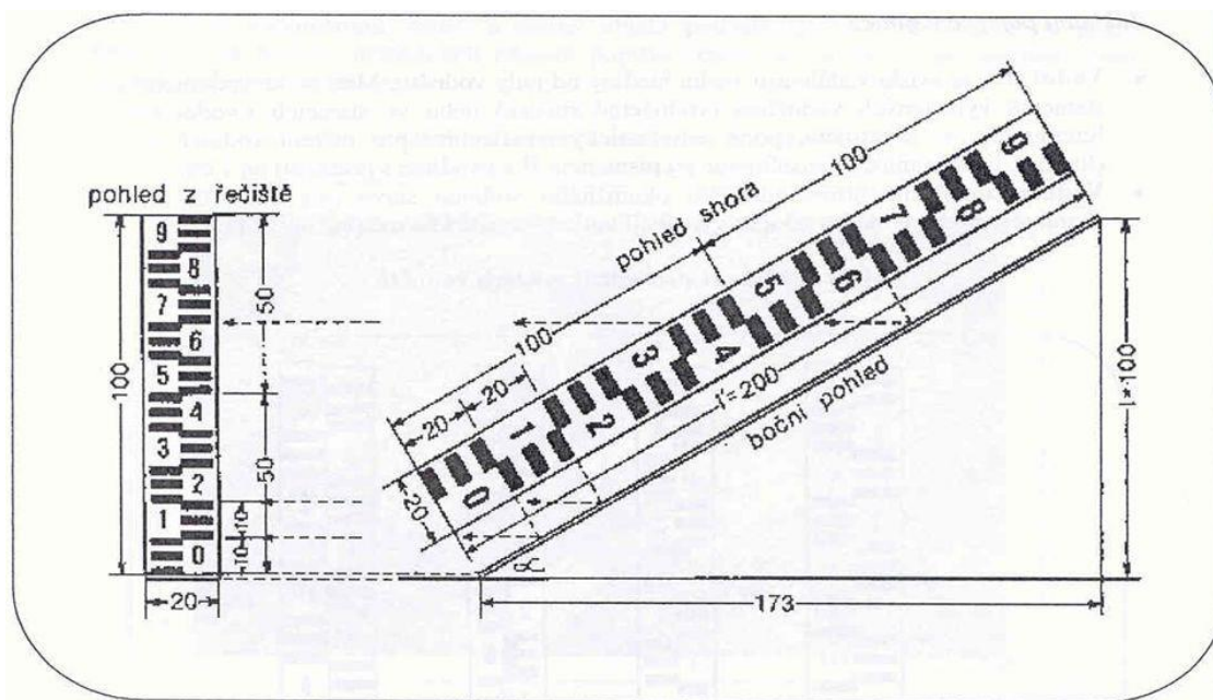
Obrázek 30 Vodočet – svislý a šikmý (zdroj Kříž a kol., 1997).
