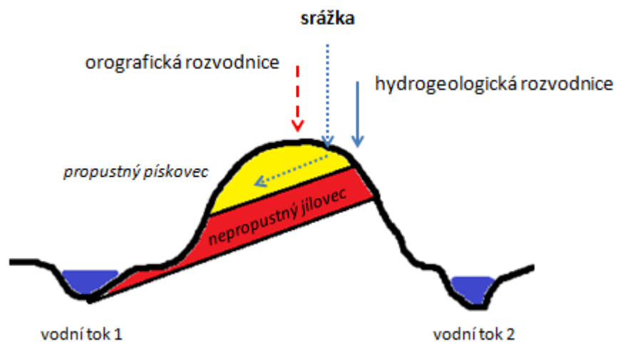
Obrázek 8 Orografická a hydrogeologická rozvodnice (vlastní zpracování).
