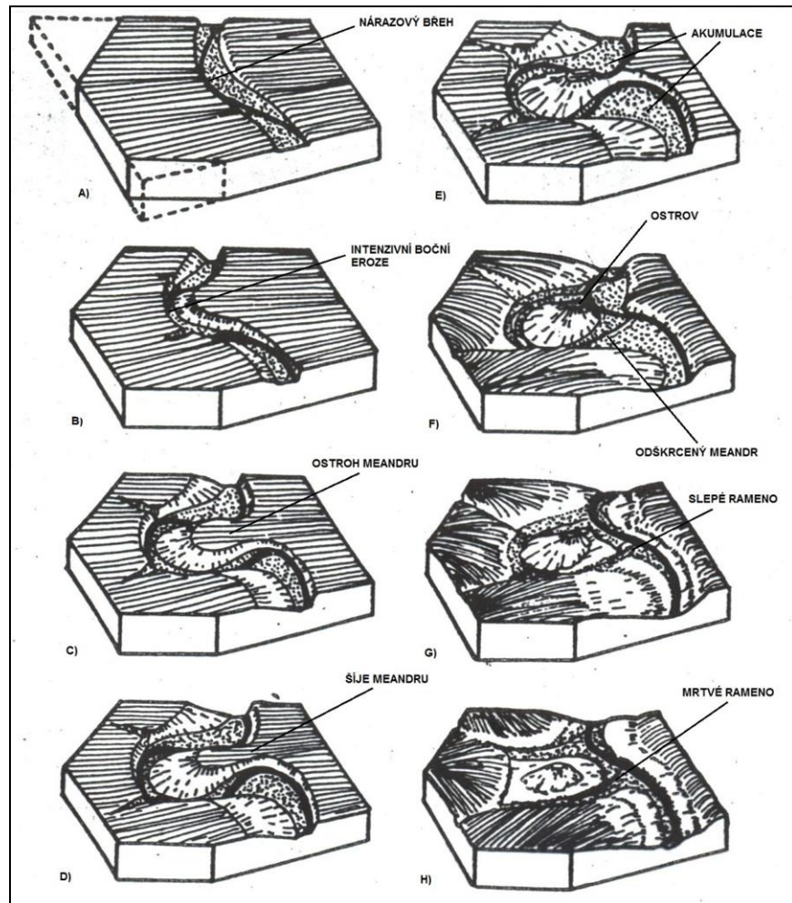
Obrázek 45 Schéma vývoje meandru (zdroj: www.rade.ic.cz, upraveno)
