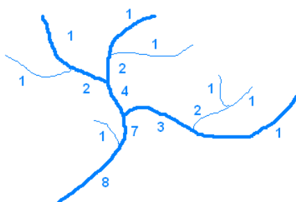
Obrázek 11 Shrevova klasifikace vodních toků (vlastní zpracování).
