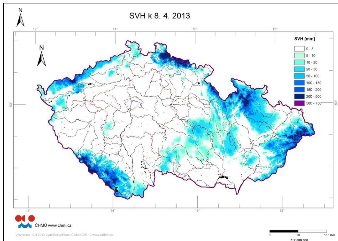
Obrázek 28 Vodní hodnota sněhu (SVH) k 8. 4. 2013 (zdroj: ČHMÚ).
