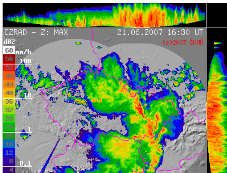
Obrázek 27 Radarový snímek území ČR se silnými bouřkami na Moravě (zdroj: ČHMÚ, Praha).
