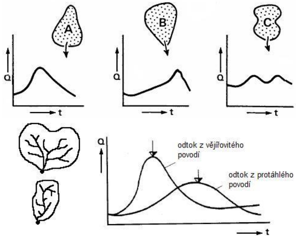
Obrázek 18 Odtok z povodí v závislosti na tvaru povodí (zdroj: alleghenygeoquest.com ; Pokorná, Zábranská 2008; upraveno autory).
