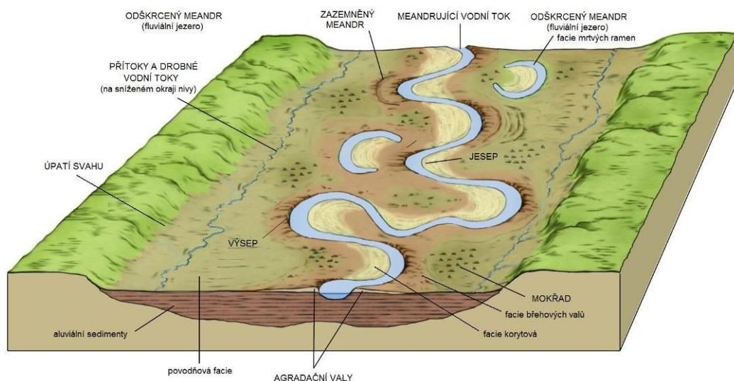
Obrázek 52 Konvexní říční niva a její části (Pearson Prentice Hall, 2005)
