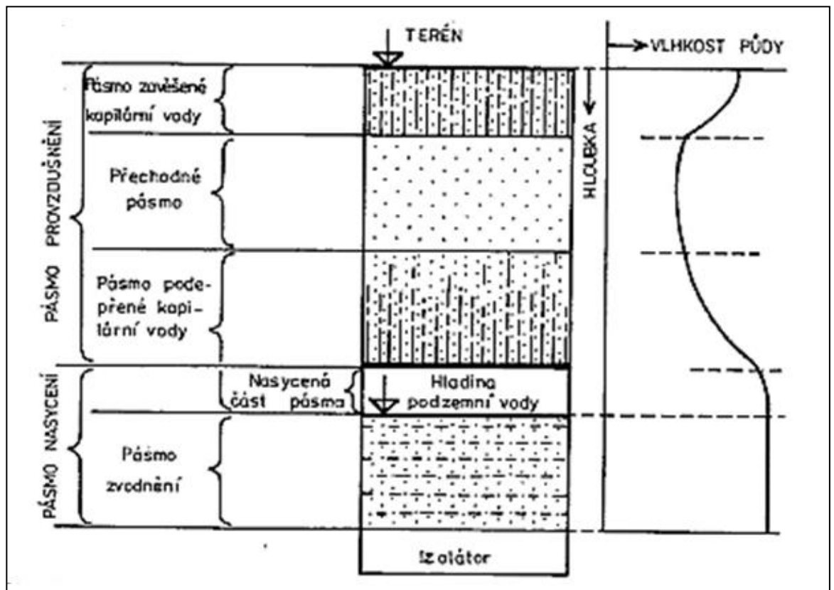
Obrázek 75 Rozdělení půdní vody v půdním a horninovém prostředí (zdroj: Tlapák, Herynek, Legát 1992)
