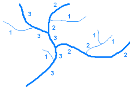
Obrázek 12 Hortonova klasifikace vodních toků (vlastní zpracování).
