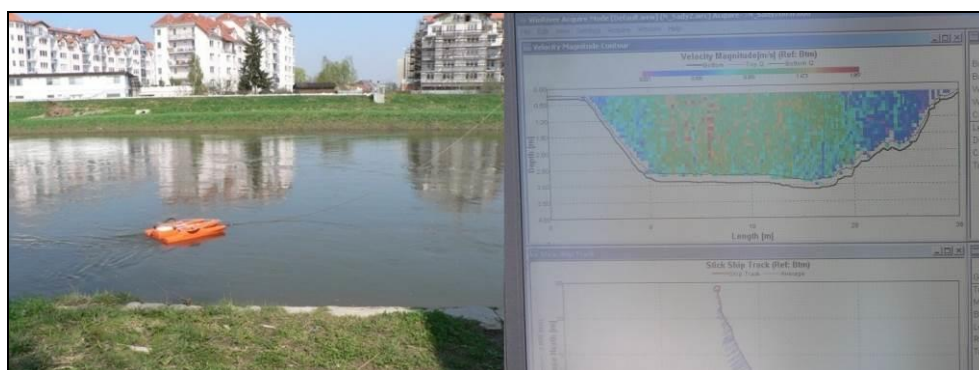
Obrázek 36 Přístroj ADCP při měření v Olomouci na Moravě a detail výstupu měření přístrojem ADCP (foto: R. Pavelková Chmelová 2010)
