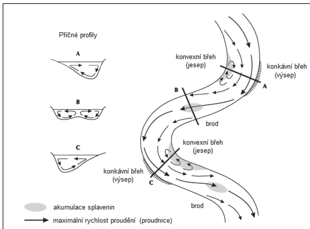
Obrázek 44 Schéma říčních zákrutů (zdroj: Huggett 2009, upraveno)
