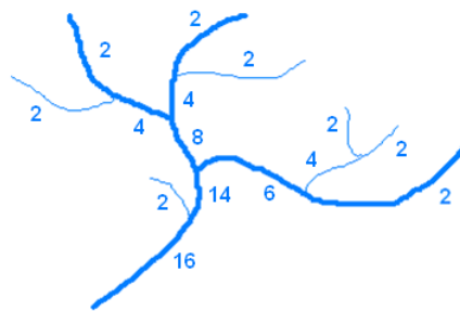
Obrázek 13 Scheiddeggerova klasifikace vodních toků (vlastní zpracování).
