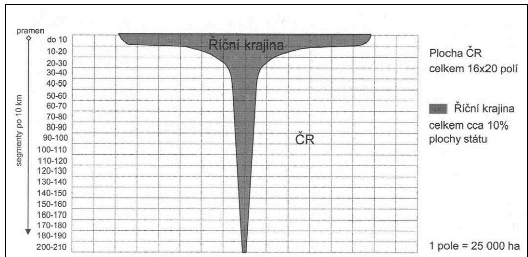
Obrázek 54 Rozložení celkové plochy říčních krajin podle vzdálenosti od pramene, ve vztahu k celkové ploše ČR (dle Štěrbý a Bednáře 2008)
