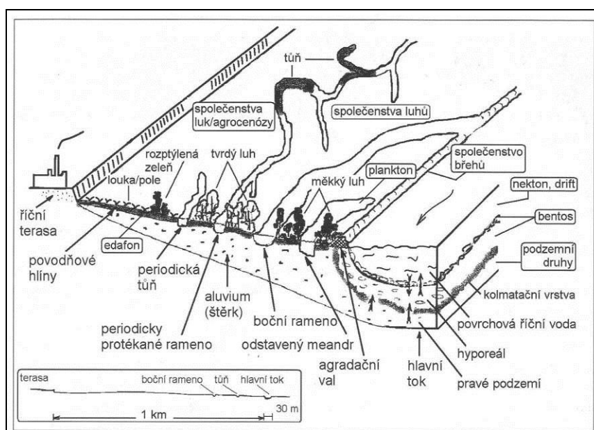
Obrázek 53 Schematický příčný řez říční krajinou (zdroj: Štěrba 2008)
