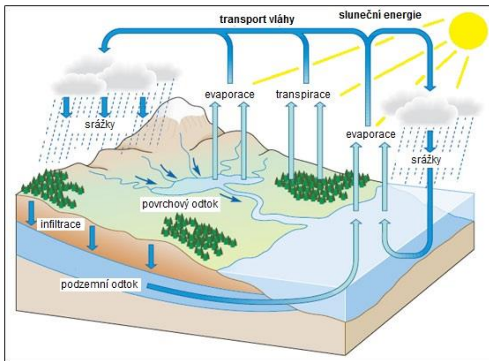
Obrázek 4 Velký oběh vody (dle Huggeta 2004, upraveno autory).
