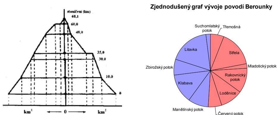
Obrázek 16 Ukázka pravoúhlého grafu vývoje povodí a kruhového (zdroj: Pokomá, Zábranská 2007; Pošta 2008).
