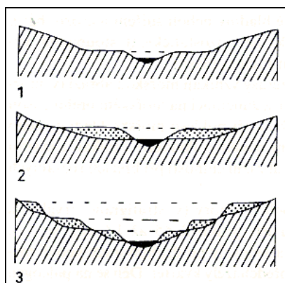
Obrázek 48 Vznik říčních teras. 1, erozní terasa ve skalním podloží; 2, akumulární říční terasa v aluviu; 3, tři terasové stupně vzniklé postupným zařezáváním toku (zdroj: www.geology.cz)
