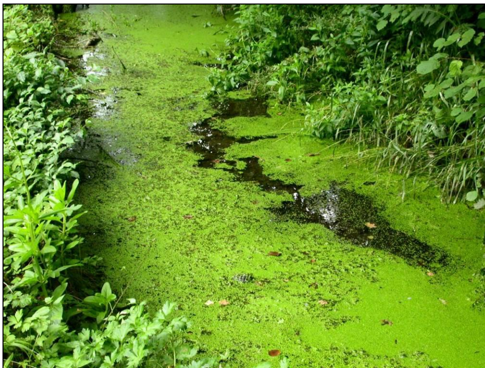
Obrázek 89 Typický projev eutrofizace – přemnožení sinic a zarůstání hladiny vodním květem (zdroj: www.wmap.cz )
