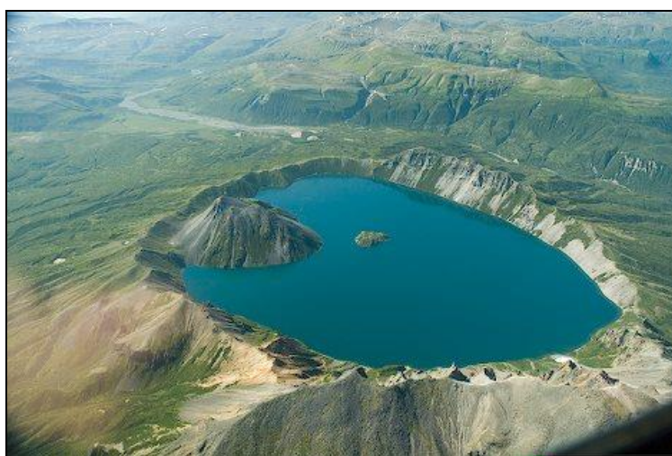
Obrázek 72 Crater Lake v USA (zdroj: www.alaska-in-pictures.com )
