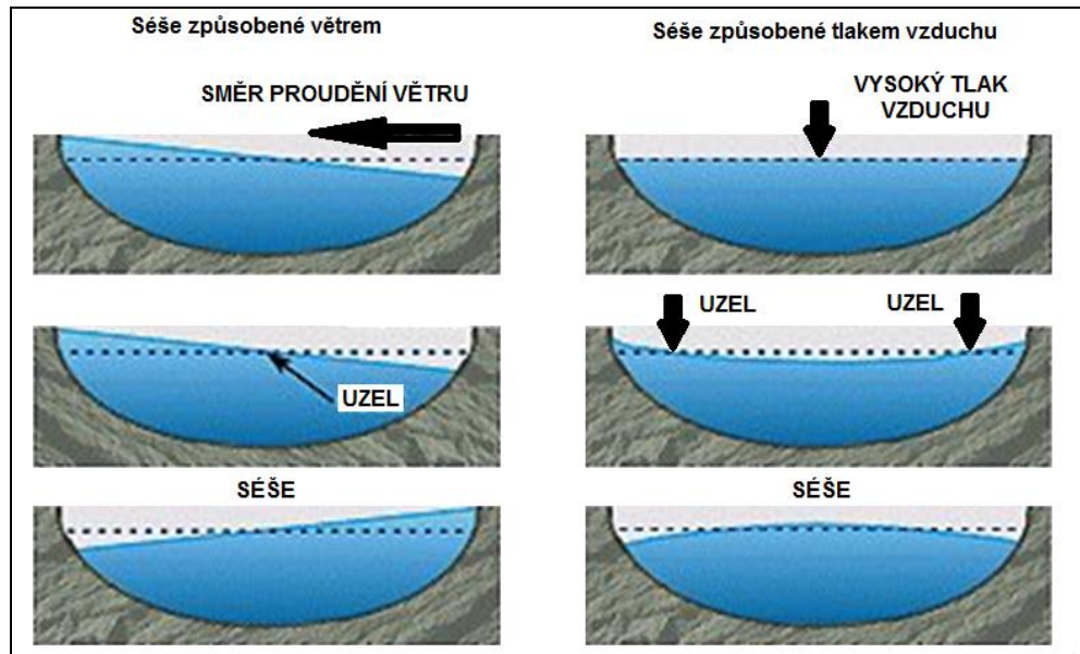
Obrázek 66 Vznik séší (seiche) – rozkývání hladiny kolem uzlových bodů (zdroj: Axler, Hagley 2004, upraveno autory)
