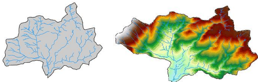
Obrázek 15 Povodí Krupé – znázornění plochy povodí z mapy (vlevo) a z digitálního modelu reliéfu. Plocha povodí stanovená planimetricky je 62,7 \text{ km}^2 , spočítaná v GIS z DMR 64,2 \text{ km}^2 . (zdroj: vlastní zpracování).
