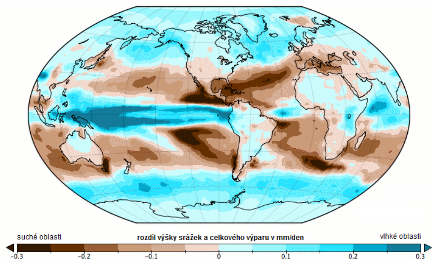
Obrázek 6 Rozdíl mezi denním úhrnem srážek a množstvím výparu. Z obrázku jasně vystupují oblasti s převažujícím výparem a tedy srážkovým deficitem (pásma pasátů) (zdroj: pme_ave_ideo.columbia.edu, upraveno autory).
