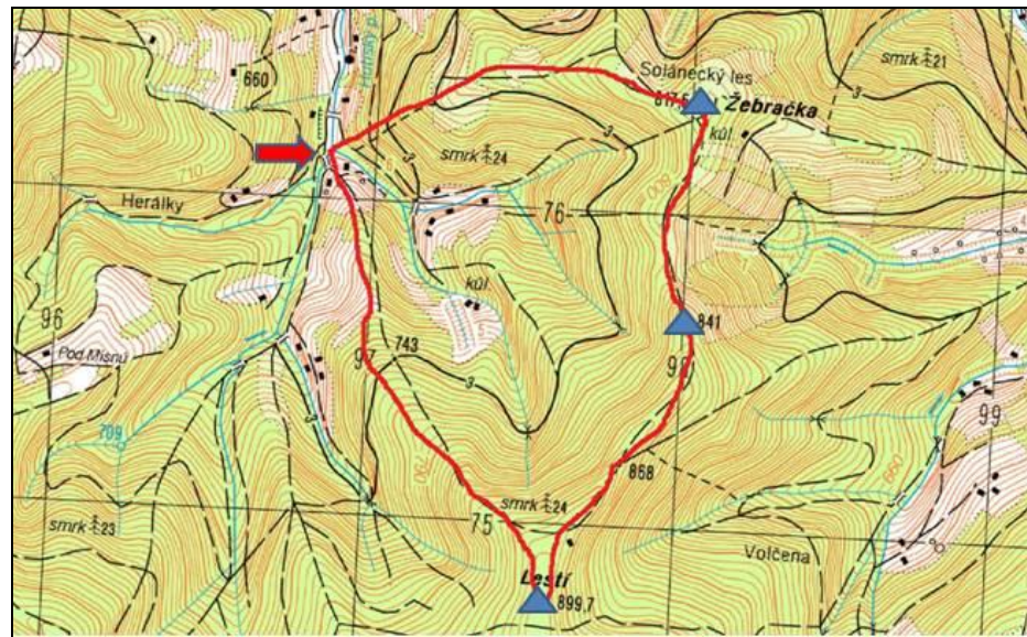
Obrázek 7 Vymezení rozvodnice (vlastní zpracování, mapový podklad CENIA).
